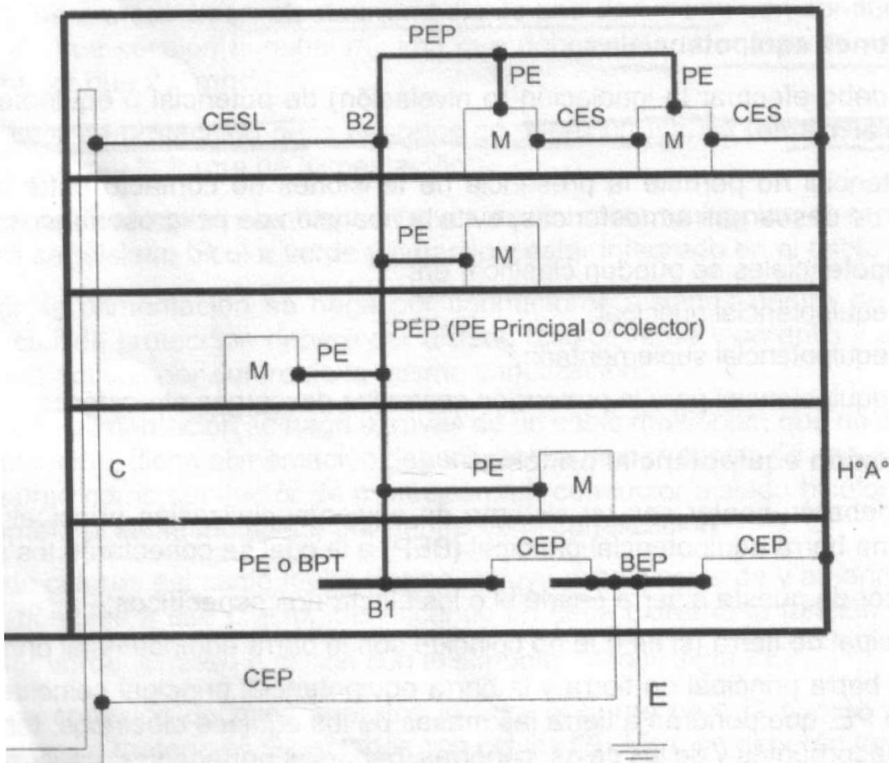
Figura 771.18.C – Ejemplo de equipotencialización
